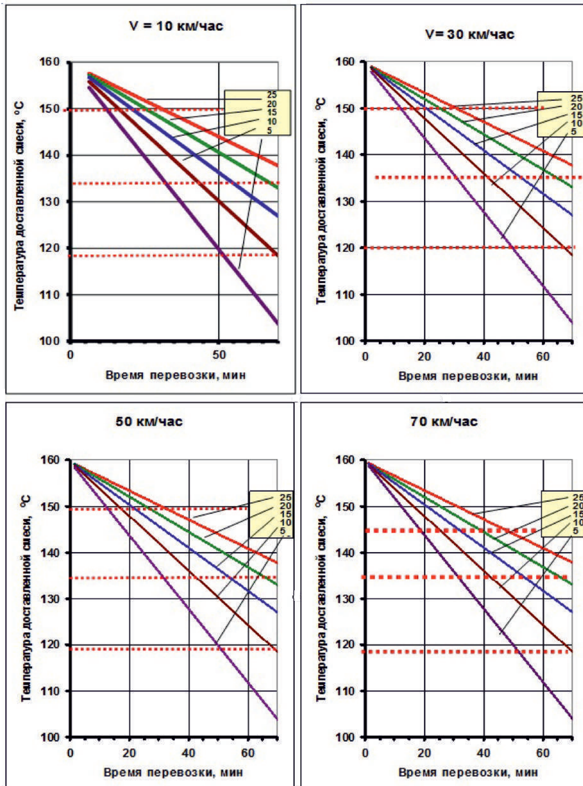
Рисунок П.1 – Время перевозки горячей асфальтобетонной смеси в автомобилях-самосвалах при температуре отгрузки t_{\text{нач}} = 160 \text{ }^{\circ}\text{C} (цифры на лучах – температура воздуха)
